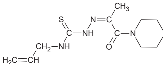
Рис. 1. Строение 4-аллилтиосемикарбазона (1-пиперидин-1-ил)пропан-1,2-диона (HL).
