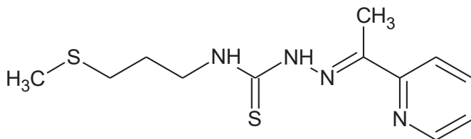
Рис. 1. Строение 4-(3-метилтиопропил)тиосемикарбазона 2-ацетилпиридина (HL).
