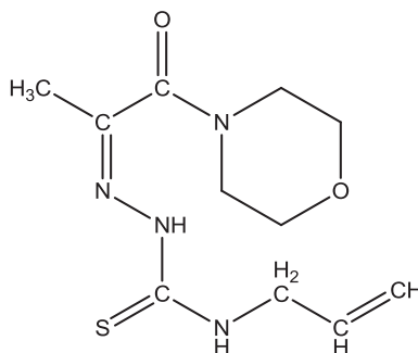
Рис. 1. Структурная формула 4-аллилтиосемикарбазона 1-(морфолин-4-ил)пропан-1,2-диона (HL).
