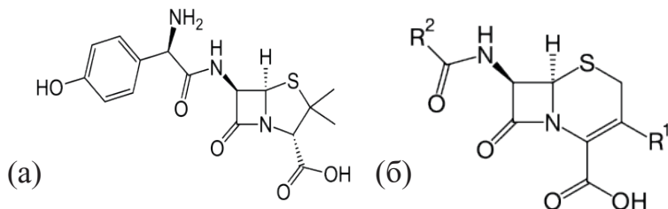
Рис. 1. Амоксициллин(а) и общая структура цефалоспоринов(б).
