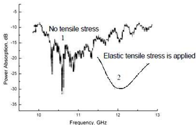
Рис.2. 1 - средние поглощающие способности экрана, содержащего микропровода с ЕФМР в микроволновых частотах в пределах от (10 - 12) ГГц для микропроводов из \text{Fe}_{68}\text{C}_4\text{B}_{16}\text{Si}_{10}\text{Mn}_2 ( R_m \sim 5 мкм, x \sim 5 ); 2 – гипотетическая кривая поглощения в случае внешнего давления
