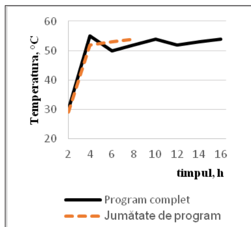
Figura 4. Variația temperaturii în interiorul sterilizatorului încărcat în funcție de timp. Condiții: [EtO] = 882 \text{ mg}\cdot\text{h/L} ; Rh = 56\%
