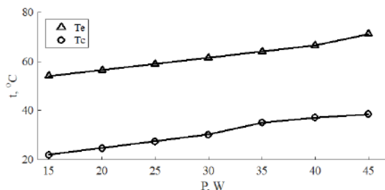
Рисунок 6. Средние стационарные температуры зон испарения и конденсации в зависимости от подводимой тепловой мощности. Количество витков – 3, рабочая жидкость – n -гексан, степень заполнения 0,7
