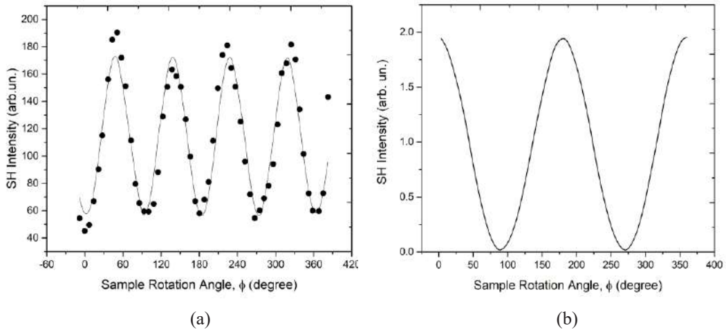
Figura 4. (a) Intensitatea semnalului AS s -polarizat generat de fasciculul fundamental s -polarizat în funcție de unghiul de rotație \varphi al eșantionului I_{ss}^{SH}(\varphi) : cerceulețe – datele experimentale; linia continuă reprezintă rezultatul calculului în baza ecuației (5). (b) Dependența intensității semnalului armonicii secunde de unghiul de rotație \varphi , calculată pentru filmul de ZnO cu textură a (ecuația (5)).
