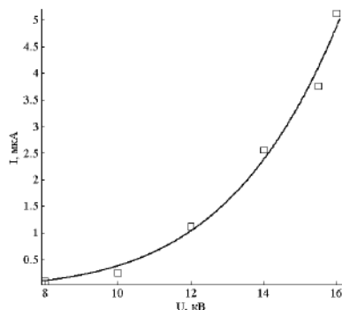
Рисунок 5. Вольтамперная характеристика ЭГД насоса
