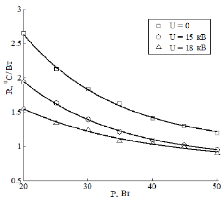
а) Термическое сопротивление
