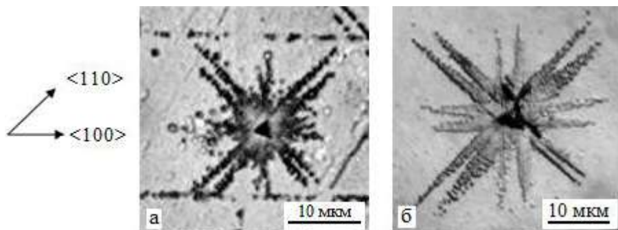
Рисунок 1. Дислокационные розетки на грани (001) монокристаллов LiF (а) и MgO (б) вокруг отпечатков индентора Берковича: а – P = 100 мН; б – P = 500 мН. Винтовые лучи расположены параллельно и перпендикулярно сторонам фотоснимков, а краевые – под 45^\circ к ним
