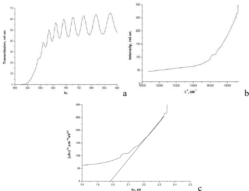
Figura 4. Spectrele de transmisie a peliculei subțiri amorphe \text{As}_{45}\text{S}_{15}\text{Se}_{40}\text{Sn}_x ( x=0 ) (a), de absorbție (b) și dependența spectrală în coordonatele lui Tauc ( E_g = 1.98 \text{ eV} ), (c). Grosimea probei d=1982 \text{ nm}
