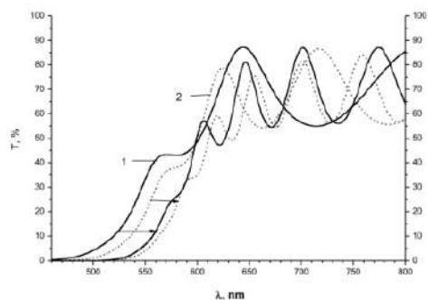
Figura 6. Spectrele de transmisie ale peliculelor subțiri amorfe (\text{As}_{45}\text{S}_{15}\text{Se}_{40})_{1-x}\text{Sn}_x cu (x=0 (1) și 0.1 (2) inițial și după expunerea cu lumina ultravioletă
