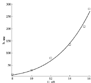
Рисунок 4. Напорная характеристика ЭГД насоса
