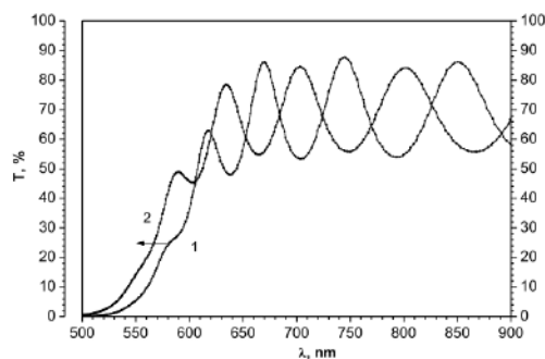
Figura 7. Spectrele de transmisie ale peliculelor subțiri amorfe \text{As}_{45}\text{S}_{15}\text{Se}_{40} , după expunerea luminii violette inițial (1) și ulterior după tratarea termică (2)
