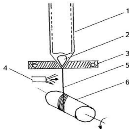
Рис. 1. Процесс литья микропровода: 1 -стеклянная трубка; 2- капля металла; 3 –индуктор; 4 –вода; 5 -микропровод со стеклянным покрытием; 6 – вращающаяся катушка для приема
