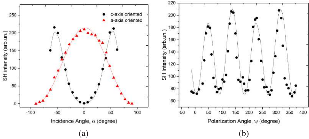
Figura 3. (a) Dependențele unghiulare I_{pp}^{SH}(\alpha) pentru filmele de ZnO orientate în direcția axelor c (cerculețe) și a (triunghiuri) depuse/w crescute pe MgO (100). Liniile continue reprezintă ajustările teoretice conform ecuațiilor (3a) și (3b).
