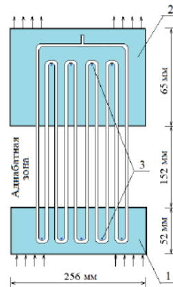
Рисунок 3. Схема ПТТ: 1 – зона испарения; 2 – зона конденсации; 3 – термодары
