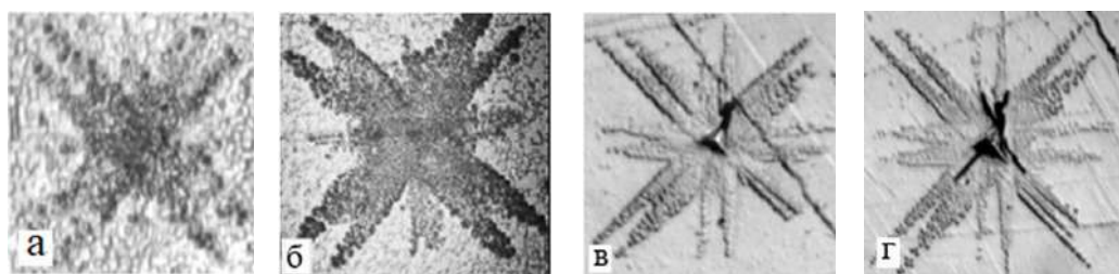
Рисунок 2. Вид дислокационных розеток на подложках LiF и MgO после снятия слоя Cu, t_1 = 85 нм. Нагрузка, P , мН: Cu/LiF: а – 200; б – 900. Cu/MgO: в – 300; г – 700. Увеличение – горизонтальная сторона каждого фотоснимка, мкм: а) – 100; б) – 220; в) – 80; г) – 120.
