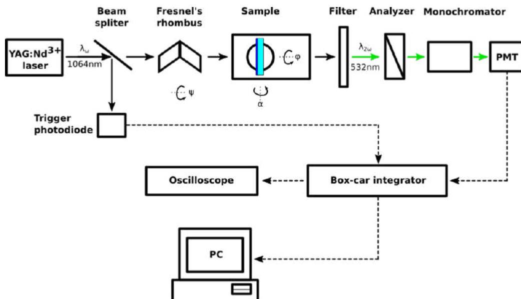
Figura 1. Schema configurației experimentale pentru măsurători ale armonicii secunde optice în transmisie
