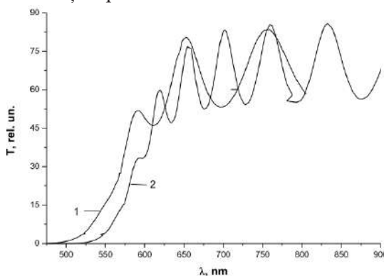
Figura 5. Spectrele de transmisie ale peliculei subțiri amorphe \text{As}_{45}\text{S}_{15}\text{Se}_{40} inițial (1) și după expunerea cu lumină ultravioletă (2)
