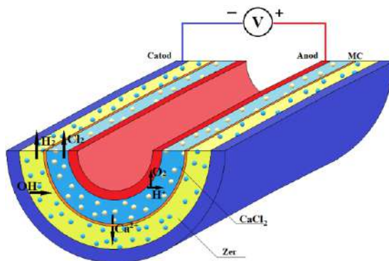
Figura 1. Schema electrolizoarelor cu carcasă semicilindrică EDC-3 și EDC-pilot [15]
