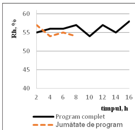
Figura 5. Variația umidității în interiorul sterilizatorului încărcat în funcție de timp. Condiții: [EtO] = 882 \text{ mg}\cdot\text{h/L} ; t = 53^\circ\text{C}
