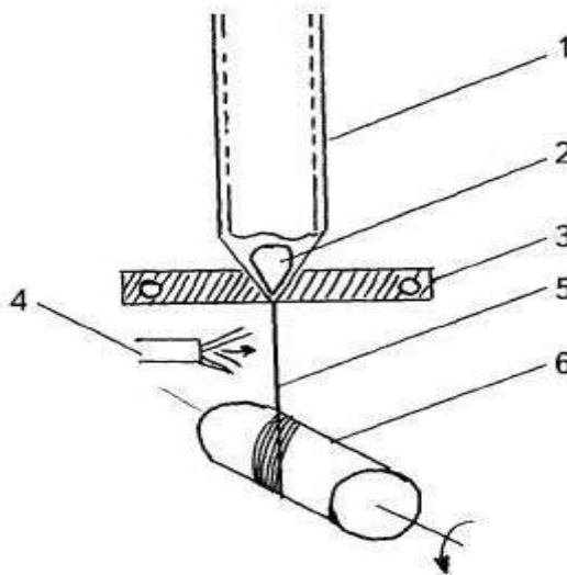
Рисунок 1. Процесс литья микропровода: 1 -стеклянная трубка; 2- капля металла; 3 –индуктор; 4 –вода; 5 -микропровод со стеклянным покрытием; 6 – вращающаяся катушка для приема
