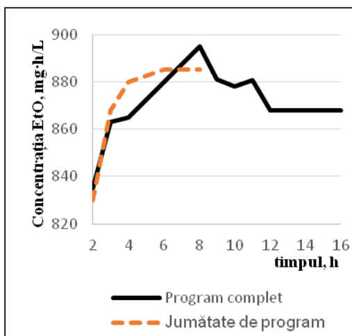
Figura 3. Variația concentrației EtO în interiorul sterilizatorului gol în funcție de timp. Condiții: t = 54^\circ\text{C} ; Rh = 56\%
