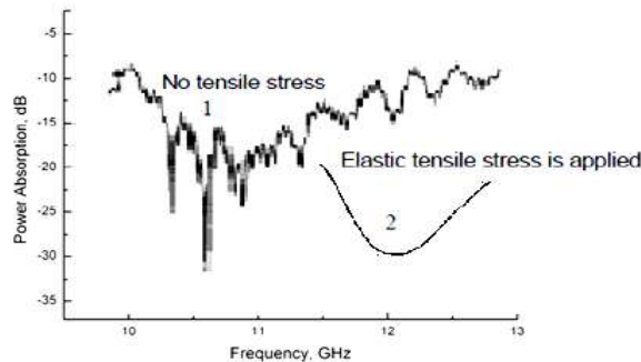
Рисунок 2. а) – средние поглощающие способности экрана, содержащего микропровода с ЕФМР в микроволновых частотах в пределах от 10 - 12 ГГц для микропроводов из Fe_{68}C_4B_{16}Si_{10}Mn_2 ( R_m \sim 5 мкм, x \sim 5 ); б) – гипотетическая кривая поглощения в случае внешнего давления
