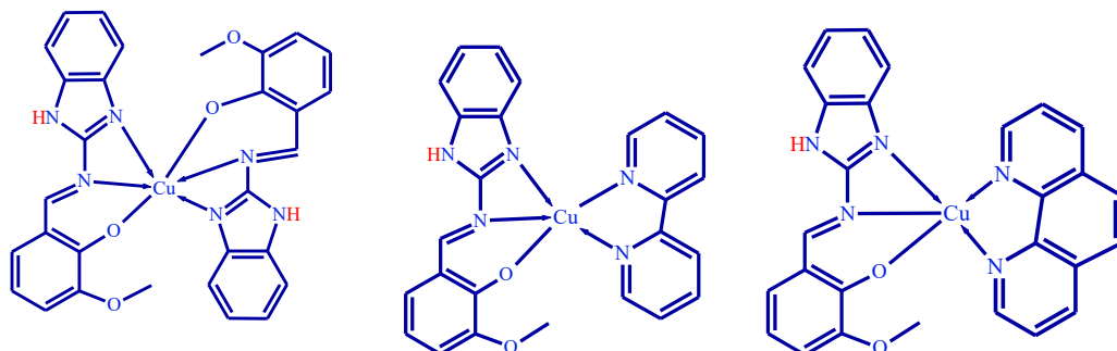
Figura 5. Formule de structură ale compușilor coordinativi de Cu(II) [4]
