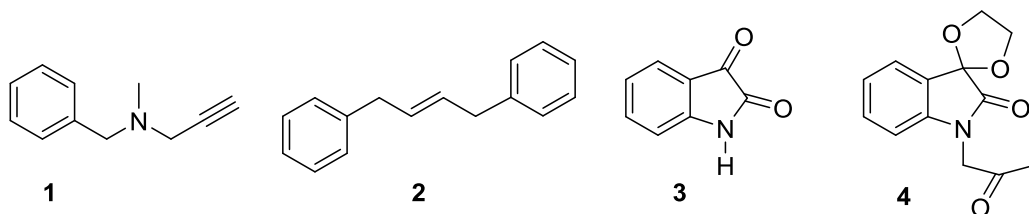
Figura 1. Inhibitori ai MAO-B: ireversibil (pargilina 1 ) și reversibili (1,4-difenil-2-butenă 2 și isatina 3 ) [7] și structura 1-(2-oxopropil)spiro[[1,3]indolin-3,2'-[1,3]dioxolan-2-onei 4
