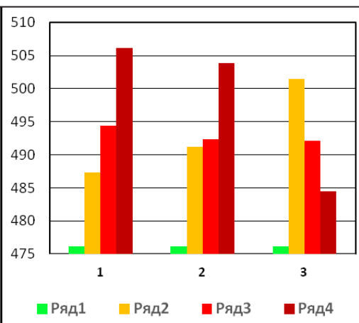
Figura 6. Valorile medii ale precipitațiilor anuale în bazinul r. Ialpug comparativ cu perioada de referință. 1- perioada 2021-2040, 2- perioada 2041-2060, 3- perioada 2081-2100. Verde- perioada de referință 1986-2005, Portocaliu- RCP2,6, Roșu-RCP4,5, Brun-RCP8,5
