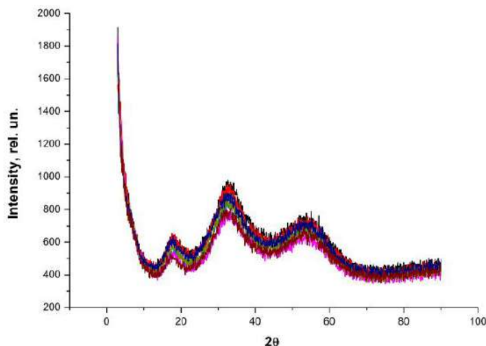
Figura 2. Măsurările difracției razelor Roentgen probelor pulbere pentru compoziția As_{45}S_{15}Se_{40})_{1-x}Sn_x ( x = 0 - 0.1 )
