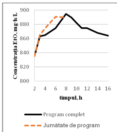
Figura 6. Variația concentrației EtO în interiorul sterilizatorului încărcat în funcție de timp. Condiții: t = 54^\circ\text{C} ; Rh = 56\%
