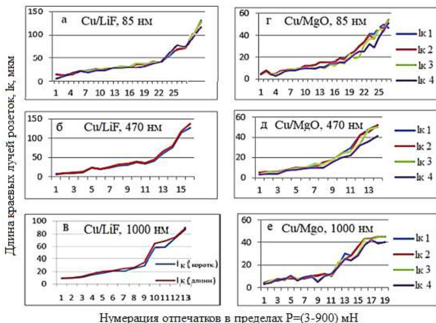
Рисунок 3. Изменение длины краевых лучей дислокационных розеток на подложках структур Cu/LiF и Cu/MgO в зависимости от величины приложенной нагрузки, P=(3-900) мН. На LiF два длинных луча близки по размерам и объединены на одну кривую, аналогично для двух коротких лучей (а). На MgO все 4 краевых луча по своим размерам отличаются друг от друга (б)
