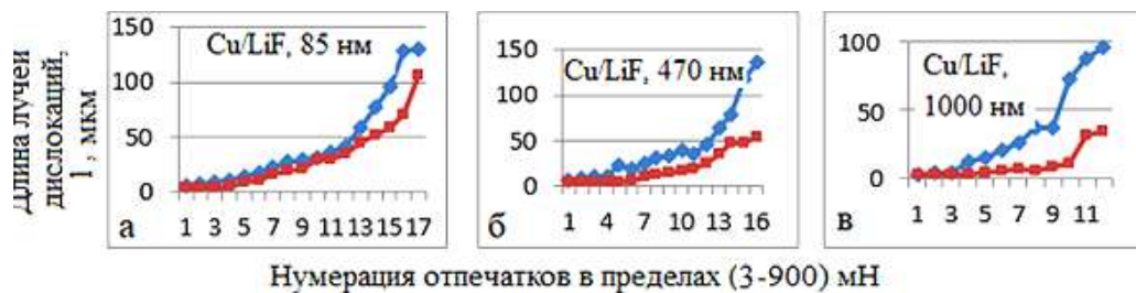
Рисунок 4. Изменение длины краевых ( l_k , синие) и винтовых ( l_v , красные) лучей дислокационных розеток на подложках структур Cu/LiF в зависимости от величины нагрузки, P=(3-900) мН
