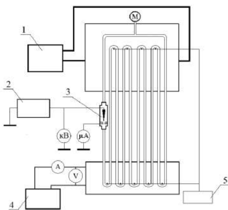
Рисунок 2. Схема экспериментального стенда: 1 – термостат; 2 – источник высокого напряжения; 3 – ЭГД насос; 4 – источник напряжения; 5 – микровольтметр
