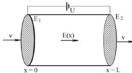
Рисунок 1. Расчётная схема ЭГД насоса
