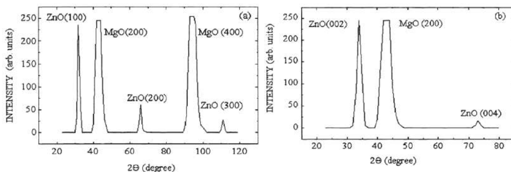
Figura 2. Difractogramele razelor X ale filmelor subțiri de ZnO depuse pe substraturi de MgO (100) încălzite la 350°C: (a) soluția precursoră – acetatul de Zn în alcool metilic, (b) soluția precursoră – acetylacetonatul de Zn în alcool metilic
