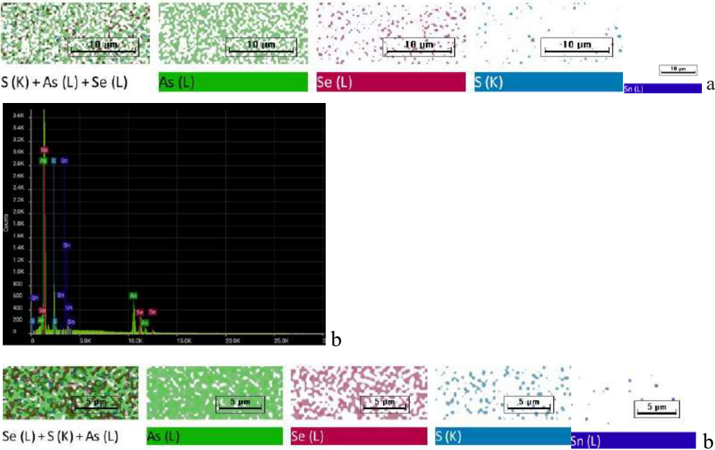
Figura 1. Imaginile și distribuția elementelor pe arie a straturilor subțiri As_{45}S_{15}Se_{40})_{1-x}Sn_x ( x=0 (a) și 0.1 (b))
