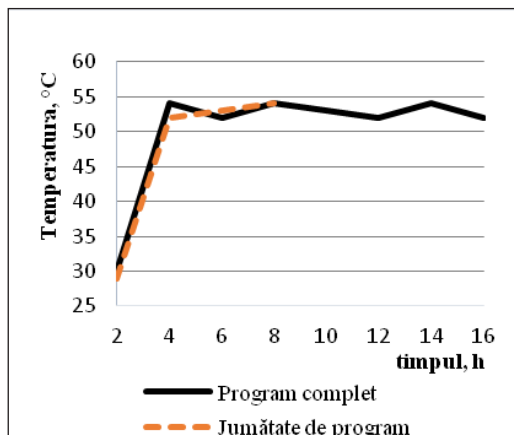
Figura 1. Variația temperaturii în interiorul sterilizatorului gol în funcție de timp. Condiții: [EtO] = 882 \text{ mg} \cdot \text{h/L} ; Rh = 56\%
