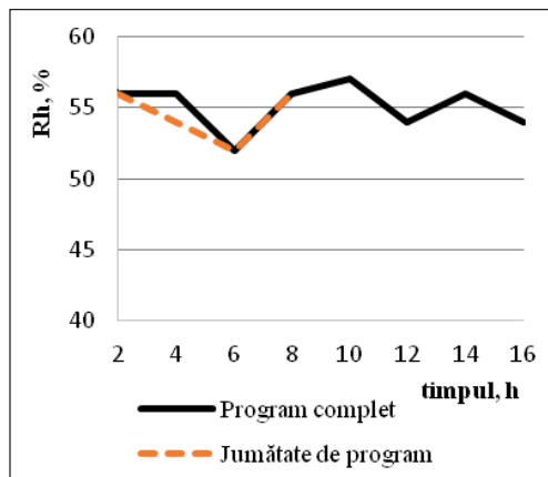
Figura 2. Variația umidității în interiorul sterilizatorului gol în funcție de timp. Condiții: [EtO] = 882 \text{ mg} \cdot \text{h/L} ; t = 53^\circ\text{C}
