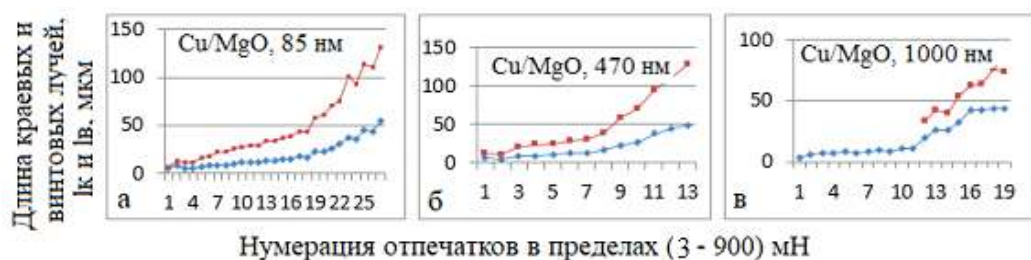
Рисунок 5. Изменение длины краевых ( l_k , красные кривые) и винтовых ( l_v , синие кривые) лучей дислокационных розеток на подложках структур Cu/MgO в зависимости от величины приложенной нагрузки, P=(3-900) мН
