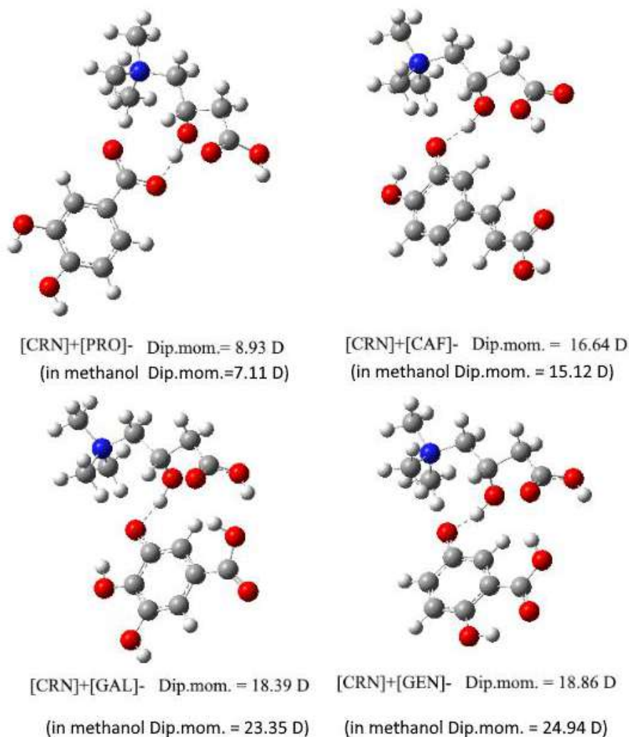
Figura 3. Geometriile optimizate și momentele dipolare calculate pentru unele perechi ionice ale lichidelor ionice studiate
