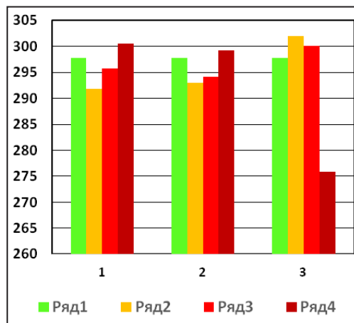
Figura 5. Valorile medii ale precipitațiilor în sezonul cald în bazinul r. Ialpug comparativ cu perioada de referință. 1- perioada 2021-2040, 2- perioada 2041-2060, 3- perioada 2081-2100. Verde- perioada de referință 1986-2005, Portocaliu- RCP2,6, Roșu- RCP4,5, Brun-RCP8,5
