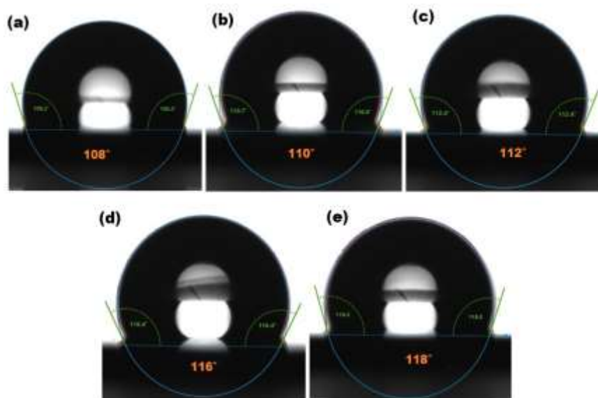
Figura 2. Umectabilitatea filmelor de CuO obținute la diferite intervale de timp: a) 5 min; b) 8 min; c) 10 min; d) 12 min și e) 15 min.
