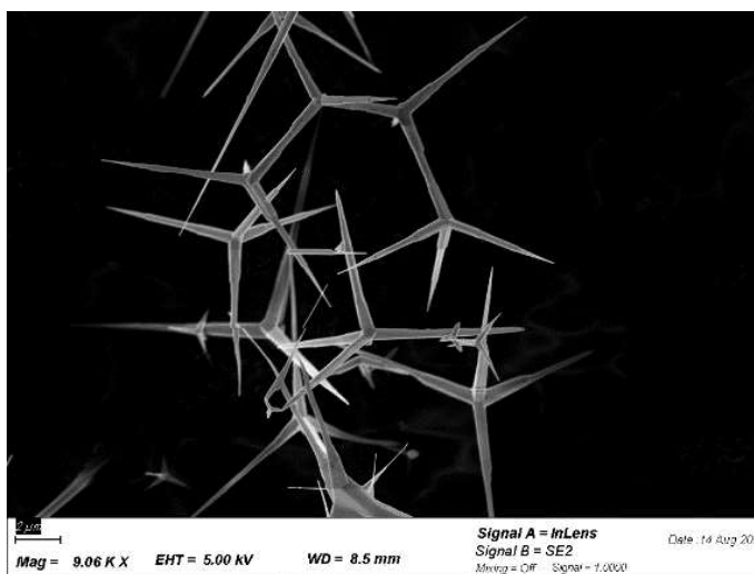
Fig. 1. SEM picture of Tetrapodal ZnO
