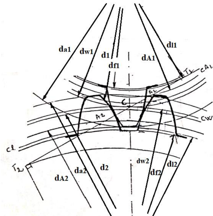
Fig. 3. Elementele geometrice ale angrenajelor [1], [2].
