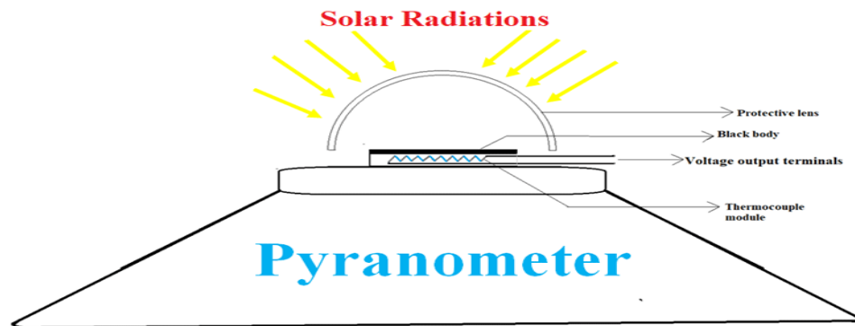
Fig. 8. Pyranometer diagram
